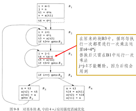
图 9-8 对基本块 B_3 中的 4 * j 应用强度消减优化
