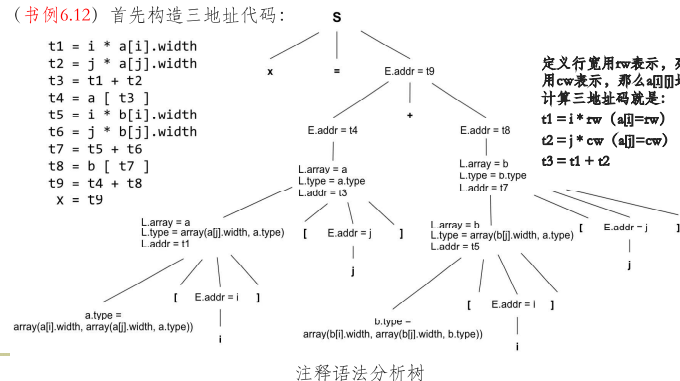
注释语法分析树
